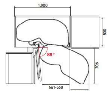
Esempio: per apertura a destra (mobile a sinistra - anta da 60 cm)
