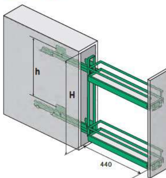
Fig.: Dimensioni in mm
