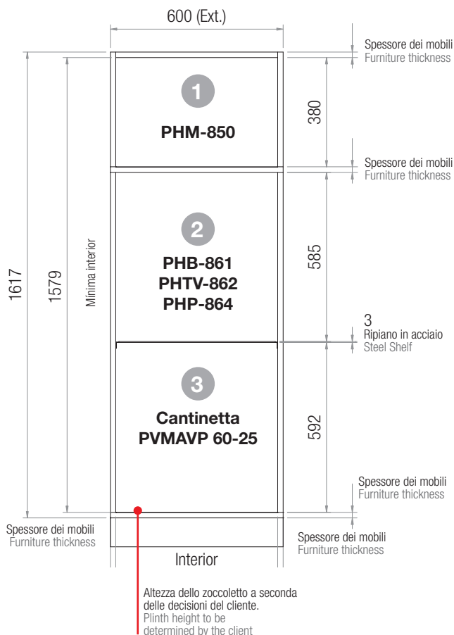
VISTA FRONTALE DEL MOBILE FRONT VIEW
